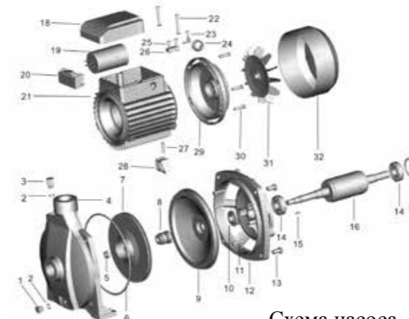
Схема насоса
